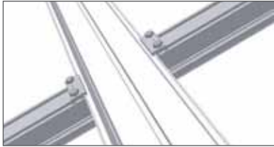
Anschluss Pfetten
