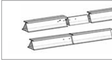
Anschluss Einschubverbinder - mit thermischer Trennung
