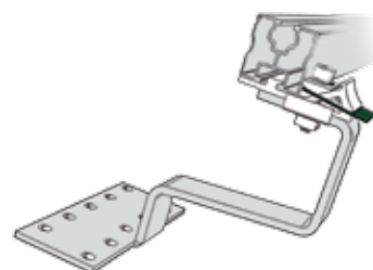
Gancio per tetto KlickTop
