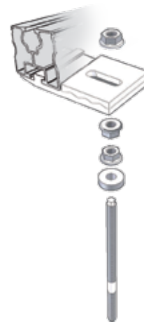
Fissaggio per tetto ondulato KlickTop
