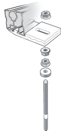
Fijación para tejado ondulado KlickTop
