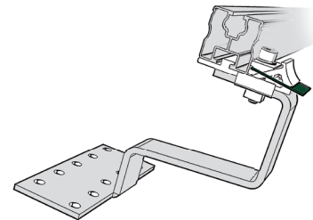
Gancho con KlickTop
