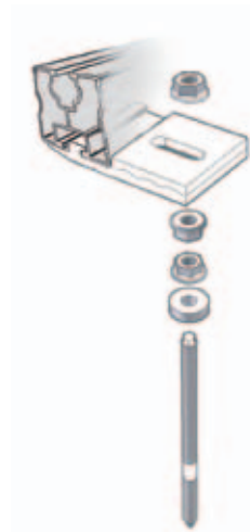
Upevnění na vlnitou střechu KlickTop
